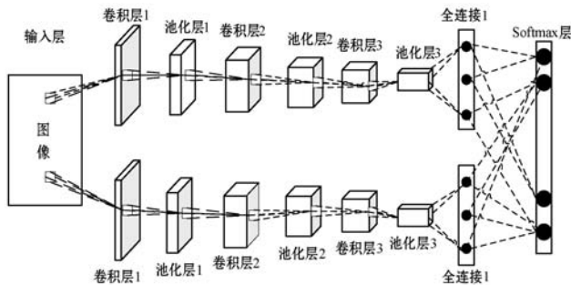
图1 卷积神经网络结构示意图
