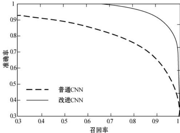
图 6 召回率曲线
