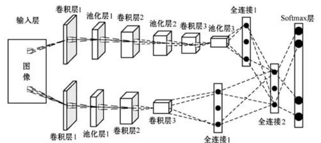
图2 改进卷积神经网络结构图
